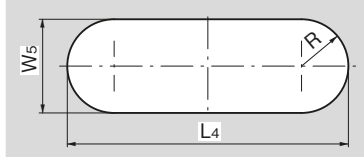
パネル穴明け寸法 Panel drilling dimensions
