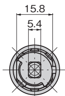
C-466-CG-CK チェンジキー Change key
