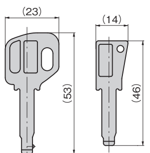
オペレーションキー Operation key チェンジキー Change key
