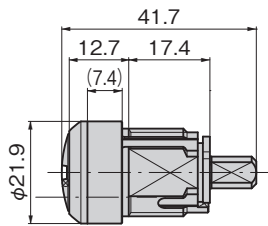
C-466-CG-RK オペレーションキー Operation key
