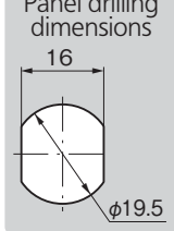
パネル穴明け寸法 Panel drilling dimensions
