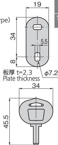
パネル穴明寸法 Panel drilling dimensions
